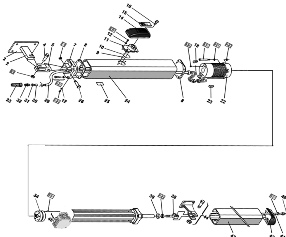
Vista esplosa
